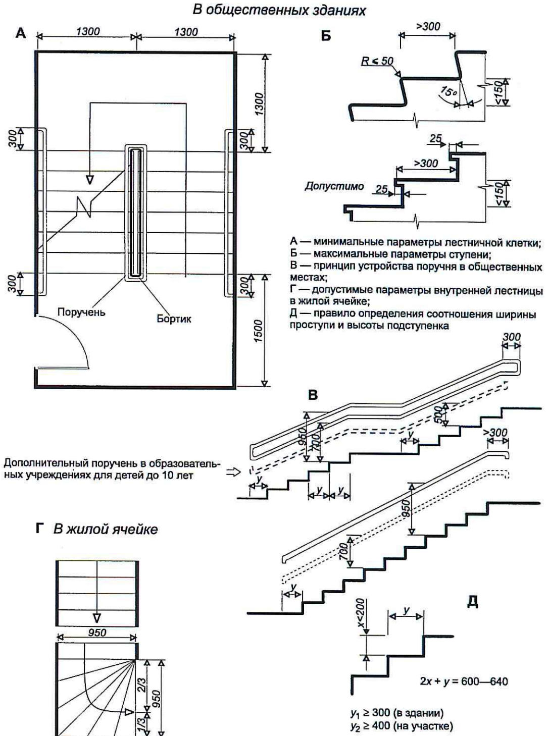
Рис. 8.7 Обустройство лестницы
