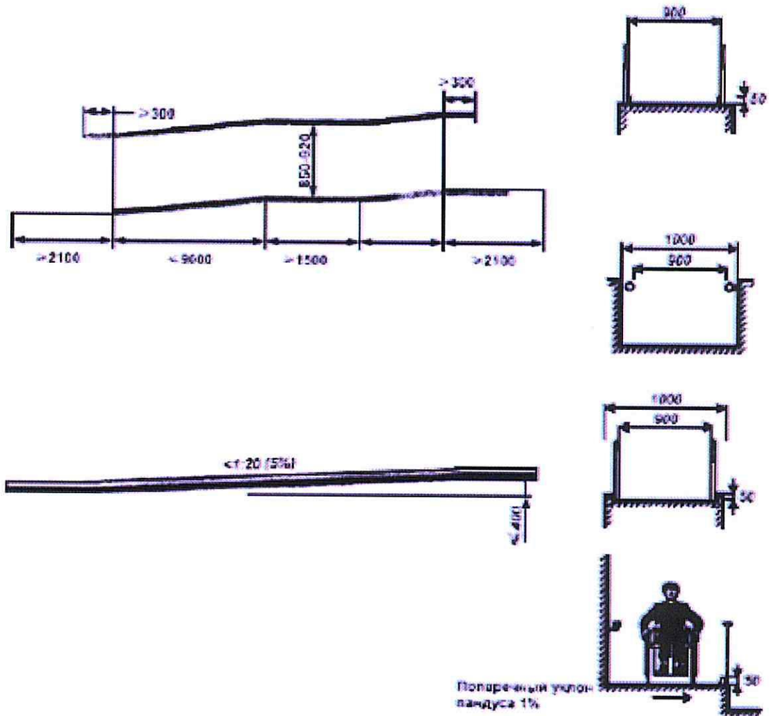
Основные параметры пандусов
