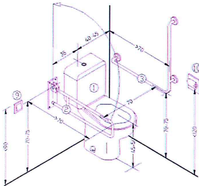
Рис. 8.12 Обустройство санитарно-бытового помещения.
