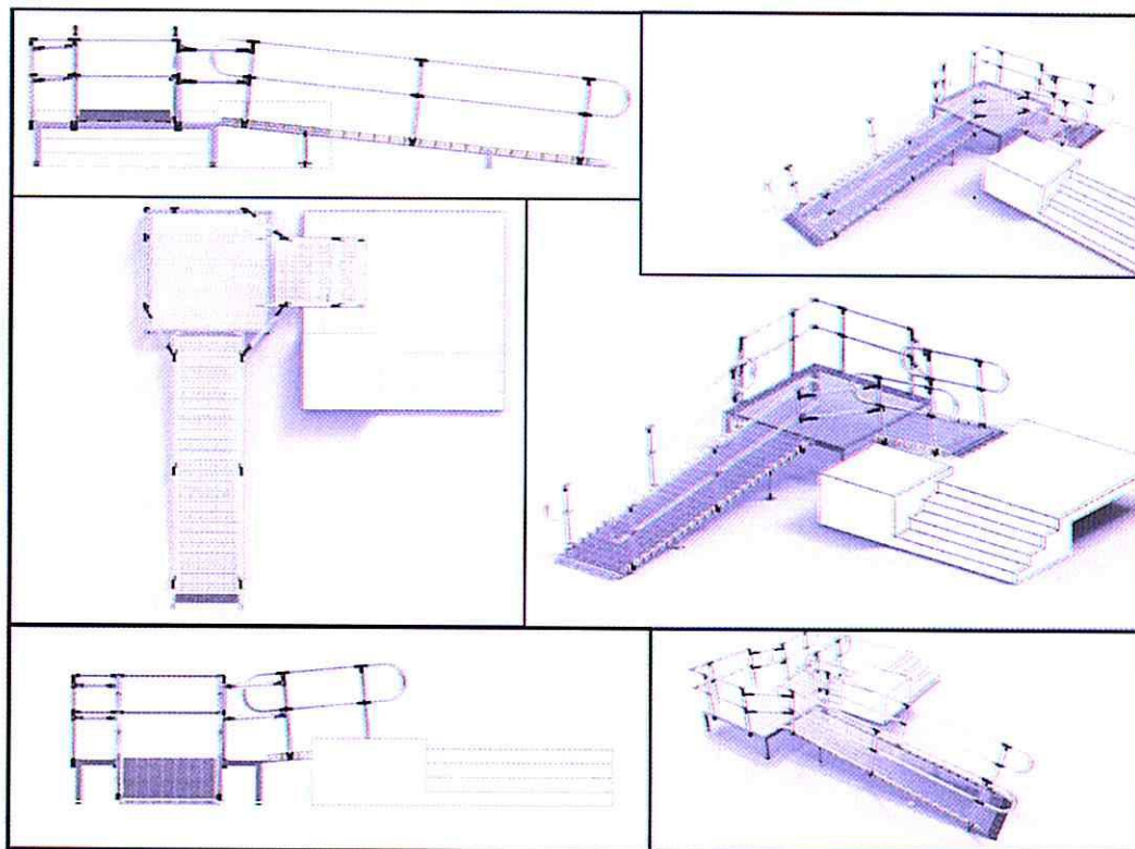
Рис. 8.10 Устройство стационарного пандуса.
