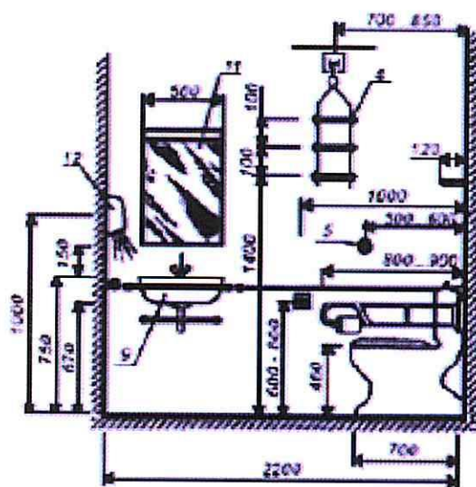
Разрез А-А
